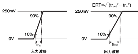
*2. 等価立上り時間 (Equivalent Rise Time)
