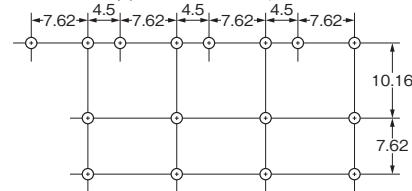
プリント基板加工寸法 (BOTTOM VIEW) 寸法公差は±0.1です
