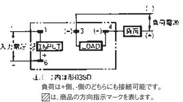
端子配置/接続 (BOTTOM VIEW)
