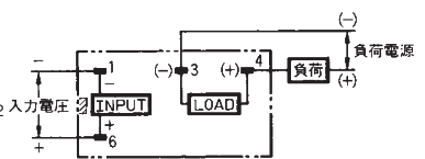
端子配置/接続 (BOTTOM VIEW)
