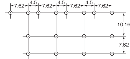
プリント基板加工寸法 (BOTTOM VIEW) 寸法公差は±0.1です
