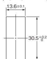
取り付け穴加工寸法 (BOTTOM VIEW)
