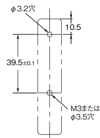
取り付け穴加工寸法
