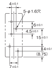
取り付け穴加工寸法 (BOTTOM VIEW)
