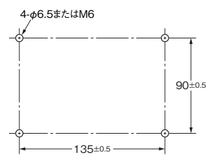
取り付け穴加工寸法
