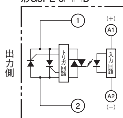
形G3PE-5□□B
