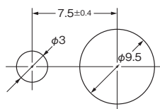
取り付け穴加工寸法
