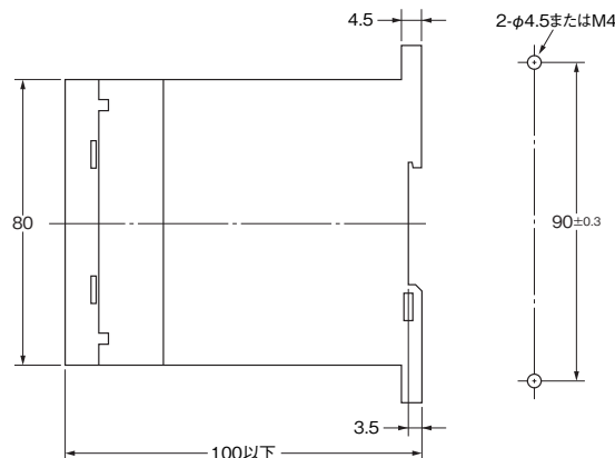
取り付け穴加工寸法
