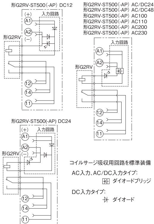
端子配置/内部接続図 (TOP VIEW)
