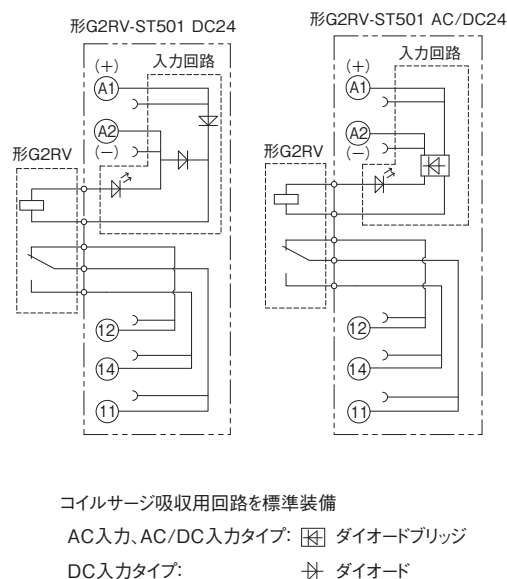
端子配置/内部接続図 (TOP VIEW)
