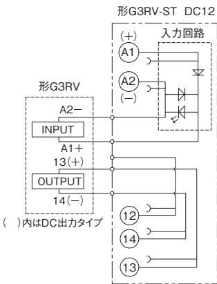
端子配置/内部接続図 (TOP VIEW)
