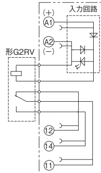
端子配置/内部接続図 (TOP VIEW)
