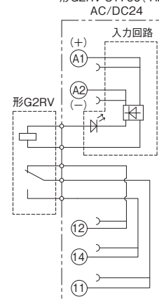
端子配置/内部接続図 (TOP VIEW)
