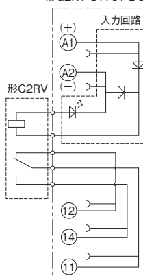
端子配置/内部接続図 (TOP VIEW)
