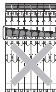
誤った取り付け 端子の浮きあり。
