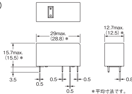
形G2RL-1-E(-ASI、-HA、-PW1)
