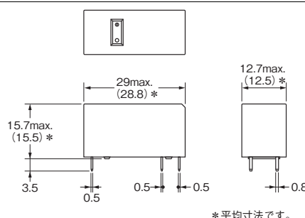
形G2RL-2A(-HA、-PW1)
