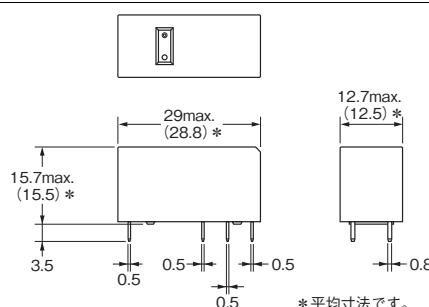
形G2RL-2(-ASI、-HA、-PW1)
