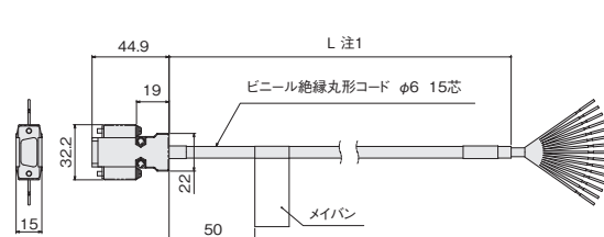
B 高輝度LED照明用パラレルケーブル
