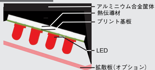
断面構造図
