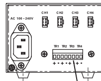
トリガ入力用端子台CH1～CH4
