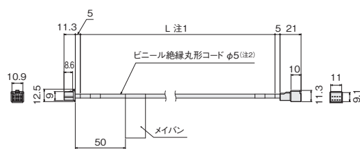
A 高輝度LED照明用延長ケーブル
