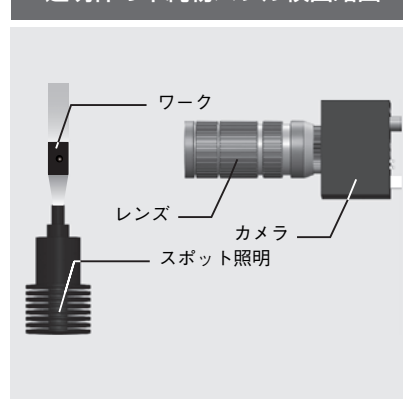
透明体の不純物バブル検出略図
