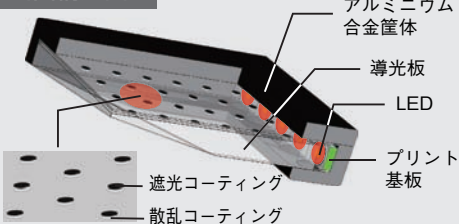
断面構造図
