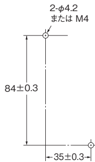
取付穴加工寸法
