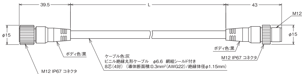
受光器用両側コネクタケーブル (別売：形F39-JD□B-D)
