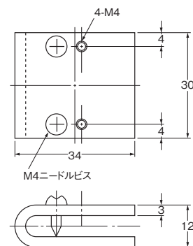
形F03-07 割シズ(ウェイト) 材質 SUS304
