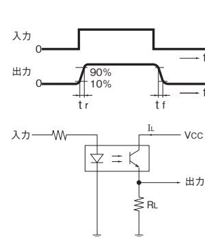
図12. 応答時間測定回路
