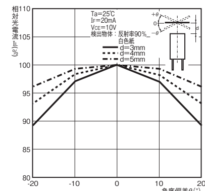
図11. 検出角度特性(TYP.)
