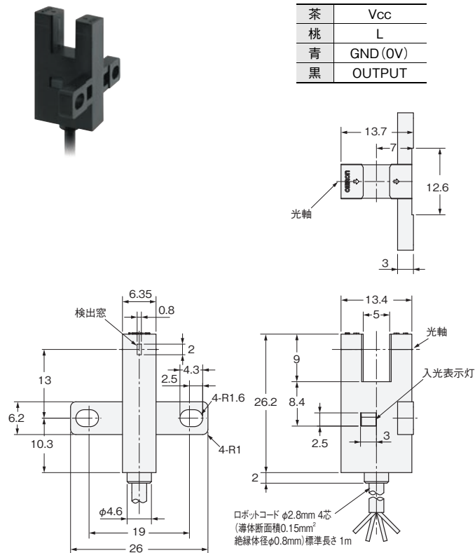
端子配置
