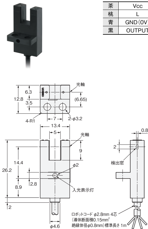
端子配置
