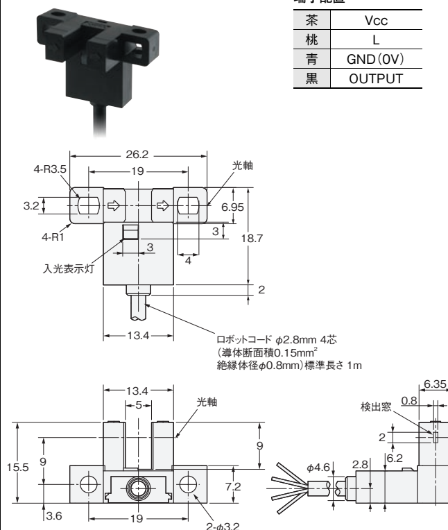
端子配置
