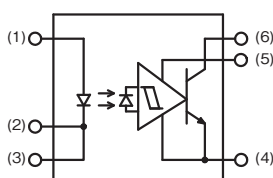
内部回路
