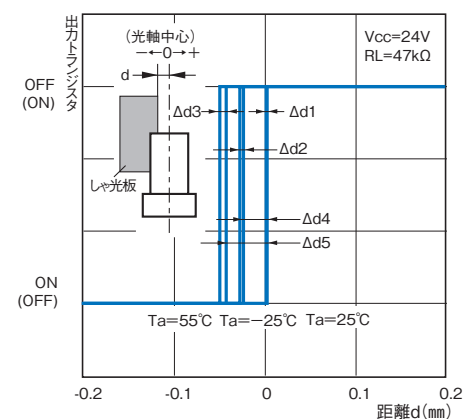
図4. 繰返し検出位置特性
