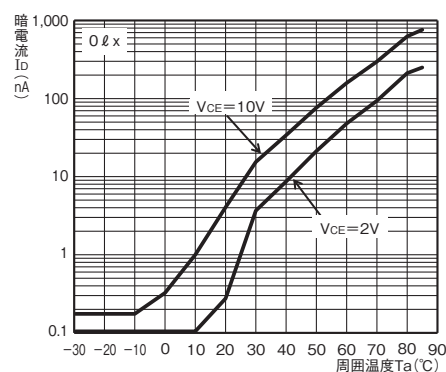
図6. 暗電流—周囲温度特性 (TYP.)
