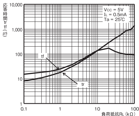
図7. 応答時間—負荷抵抗特性 (TYP.)
