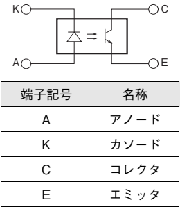
内部回路
