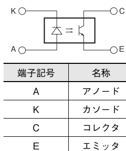
内部回路
