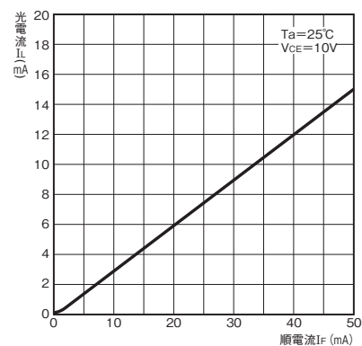
図3. 光電流—順電流特性 (TYP.) EE-SV3(-B)
