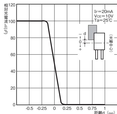
図10. 検出位置特性 (TYP.) EE-SV3-G(S)
