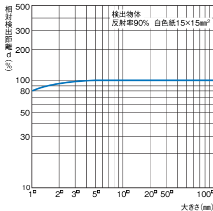
形EE-SPY□□□
