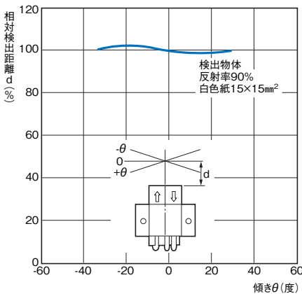
形EE-SPY312/412
