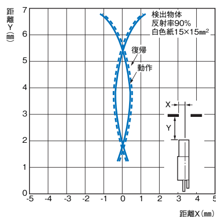
形EE-SPY312/412
