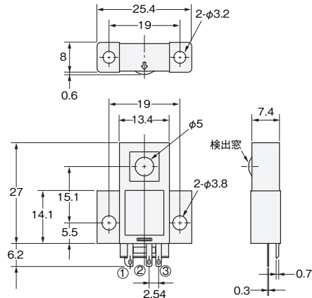
端子配置
