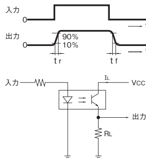
図11. 応答時間測定回路
