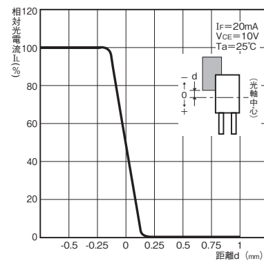
図9. 検出位置特性(TYP.) EE-SJ3-G
