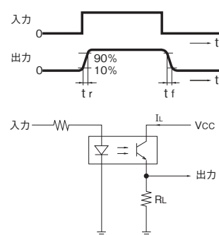
図12. 応答時間測定回路
