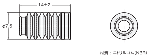
形E9NC-G5
