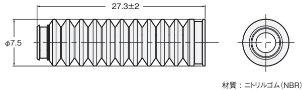
形E9NC-G12
