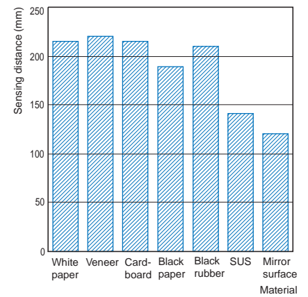
E3ZM-LS□4H(LS□9H)
