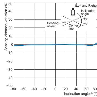
E3ZM-LS□2H(LS□7H)
