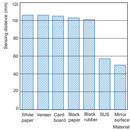
E3ZM-LS□1H(LS□6H)
