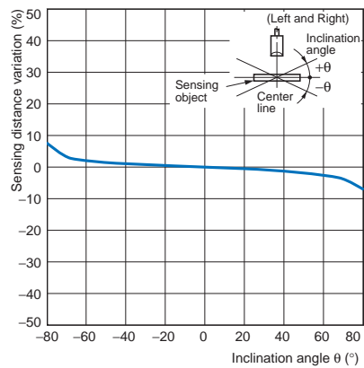
E3ZM-LS□1H(LS□6H)
