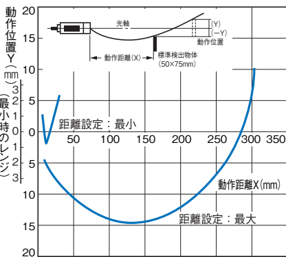
形E3S-LS20XE4
