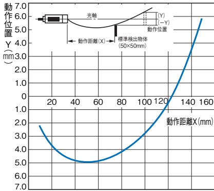
形E3S-LS10XE4
