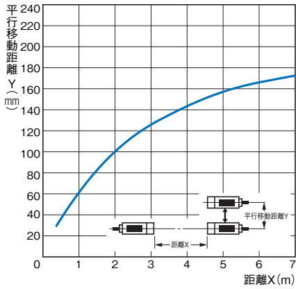
形E3S-5E4 (41)
