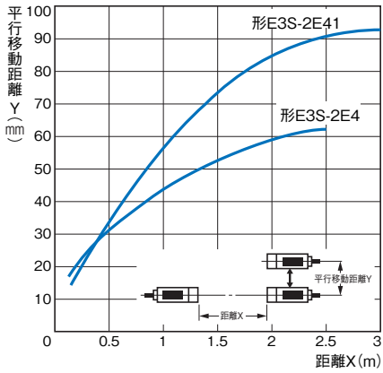
形E3S-2E4 (41)
