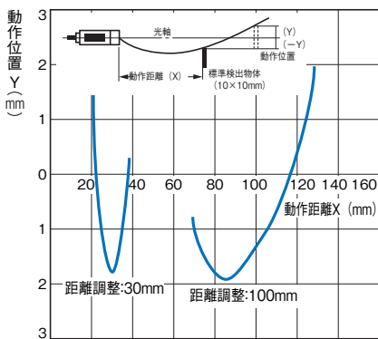
形E3S-LS10XE4
