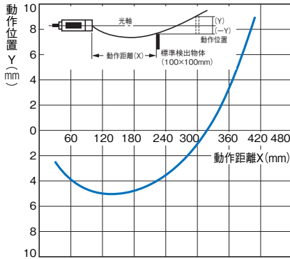
形E3S-LS20XE4
