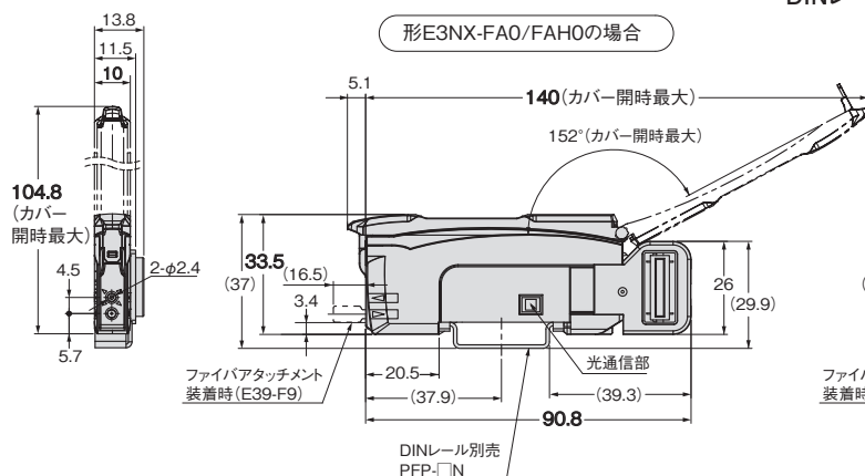
DINレール装着時
