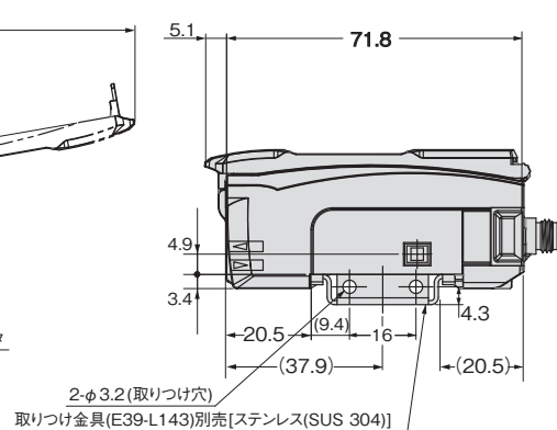
取り付け金具装着時
