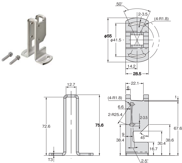
形E39-L214
