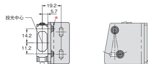
センサ装着時の寸法 (例：形E3AS-F1500□)
