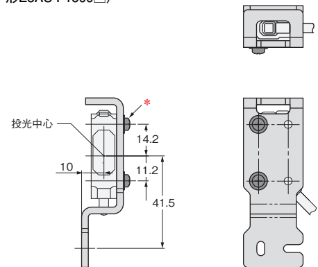
センサ装着時の寸法 (例：形E3AS-F1500□)
