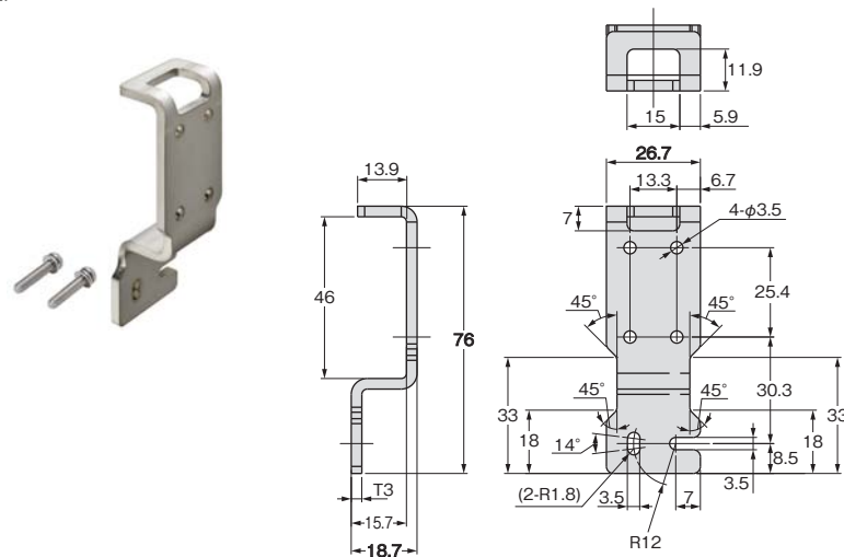
センサ装着時の寸法 (例：形E3AS-F1500□)
