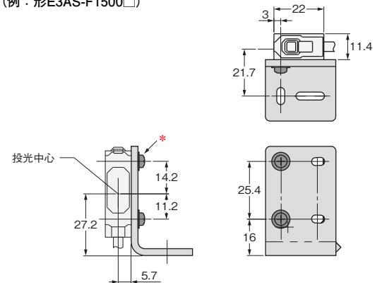
センサ装着時の寸法 (例：形E3AS-F1500□)
