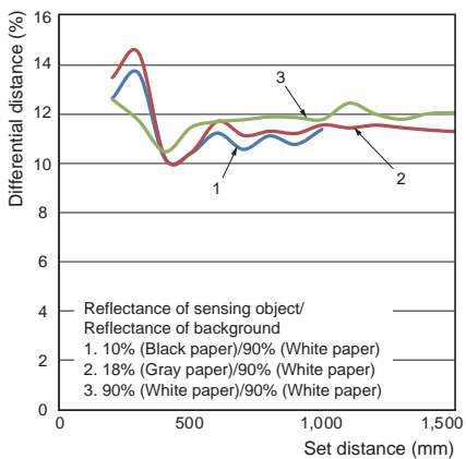
E3AS-F1500□
