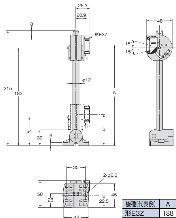
形E39-L93FH
