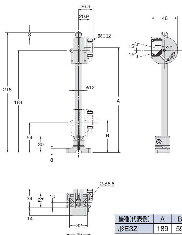
形E39-L93H
