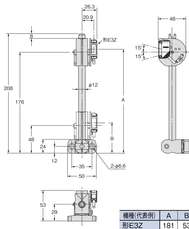
形E39-L93FV
