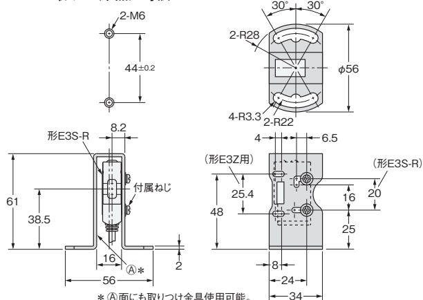
形E39-L98
