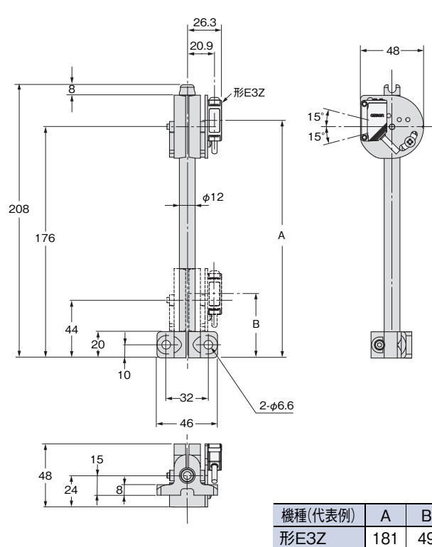
形E39-L93V
