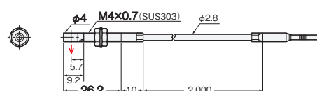
33-I E32-T61-S 2M (カット不可) + E39-F2
