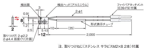
(19-F) E32-D25ZR 2M (フリーカット)
