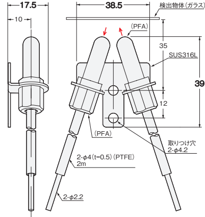
(59-H) E32-L11FS 2M (フリーカット)
