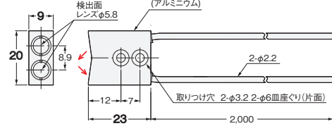
(59-F) E32-A09H2 2M (カット不可)
