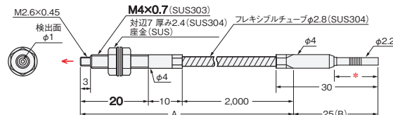
49-G E32-T61-S 2M (カット不可)
