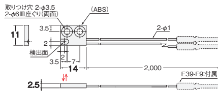
④1-A E32-L24S 2M (フリーカット)
