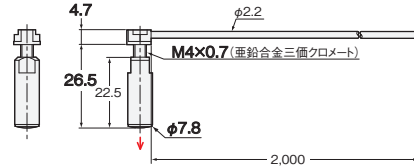
31-D E32-T11N 2M (フリーカット) + E39-F16
