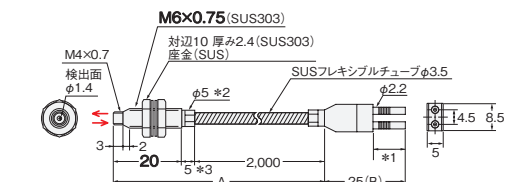
51-I E32-D61-S 2M (カット不可)
