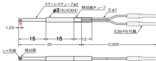
(23-A) E32-D24R 2M (フリーカット)
