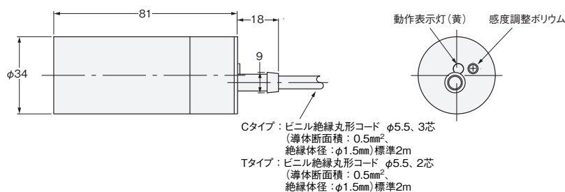
形E2K-C20M□□
