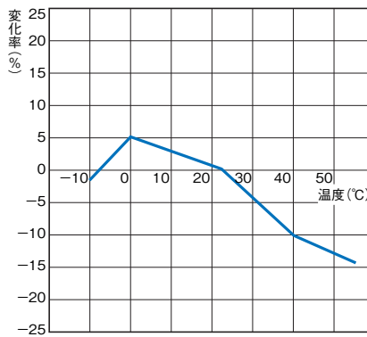
形E2J-W20MA
