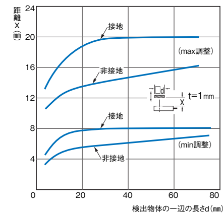
形E2J-W20MA
