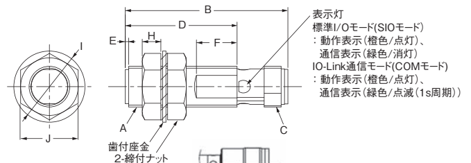
形E2EQ-X□8-M1タイプ: コネクタ部形状
