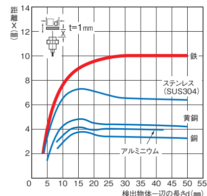
形E2EQ-X10D1 (-M1 (T) GJ)
