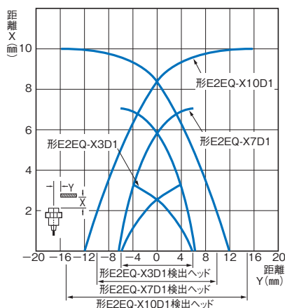
形E2EQ-X□D□ (-M1 (T) GJ)
