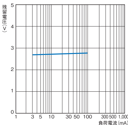
形E2EQ-X□D□ (-M1 (T) GJ)
