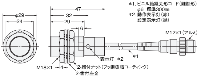
形E2EQ-X7D1-M1 (T) GJ
