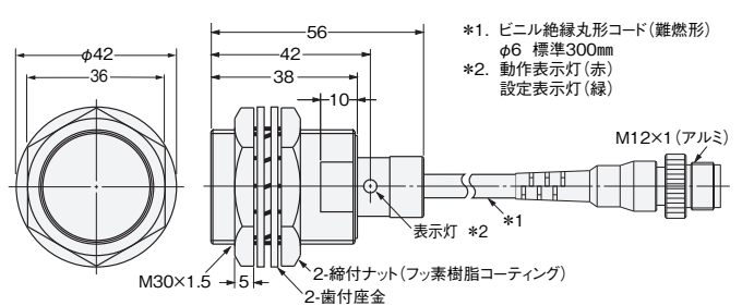
形E2EQ-X10D1-M1 (T) GJ
