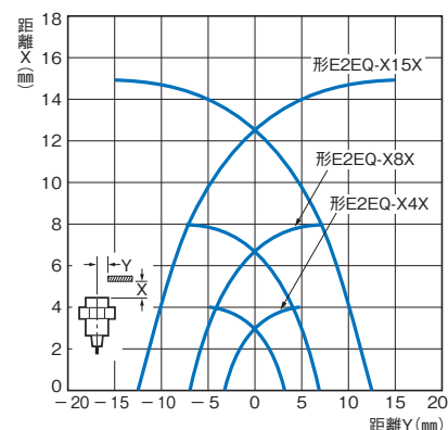
形E2EQ-X□X□ (-M1 (T) J)
