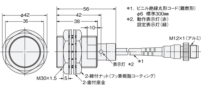
形E2EQ-X10D1-M1 (T) GJ
