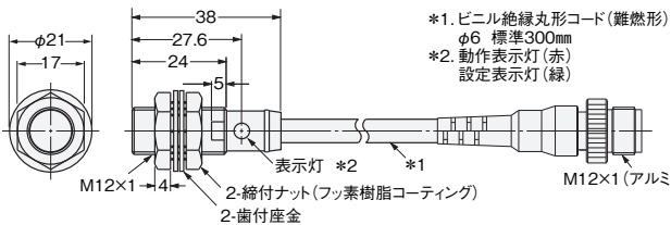
形E2EQ-X3D1-M1 (T) GJ
