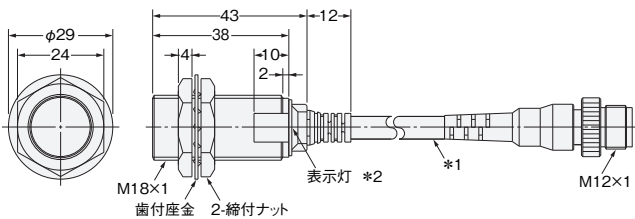
形E2EQ-X8X1-M1 (T) J
