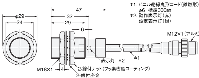
形E2EQ-X7D1-M1 (T) GJ
