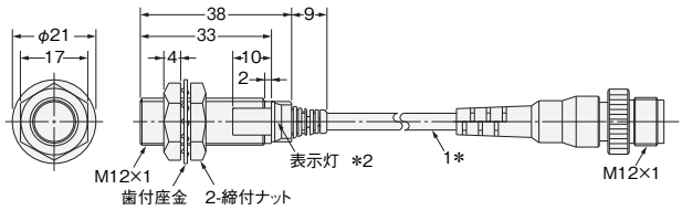
形E2EQ-X4X1-M1 (T) J
