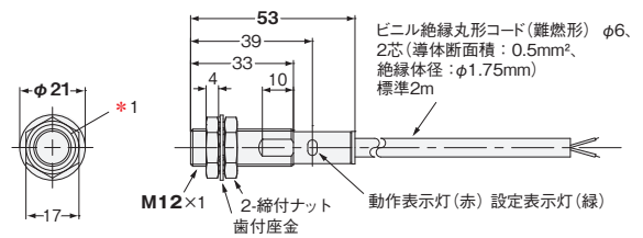
形E2EF-X3D1 -QX3D1
