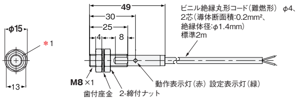
形E2EF-X2D1 -QX2D1
