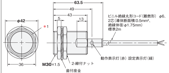
形E2EF-X12D1 -QX12D1
