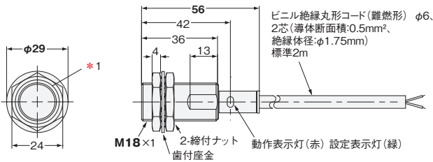
形E2EF-X7D1 -QX7D1
