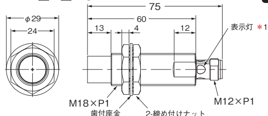
形E2E-X40M□L30-M1
