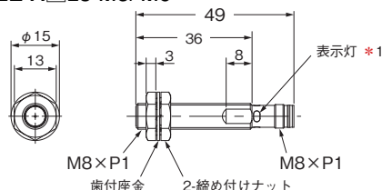
形E2E-X□L8-M1
