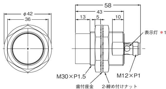
形E2E-X20MD□-M1/-M1G
