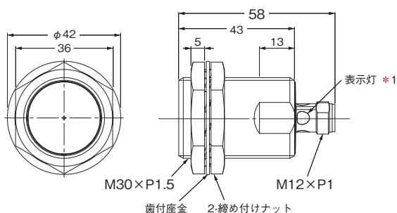
形E2E-X10D□-M1/-M1G
