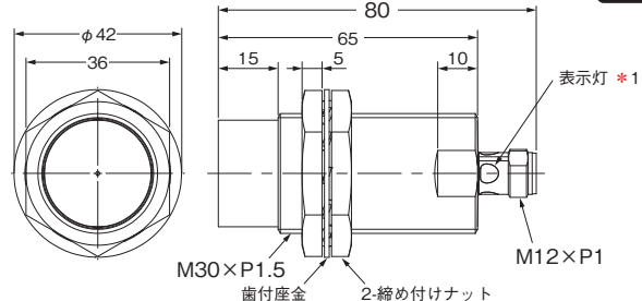
形E2E-X50M□L30-M1
