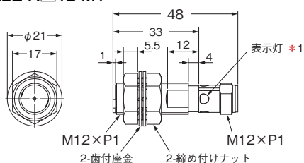
形E2E-X□18-M1
