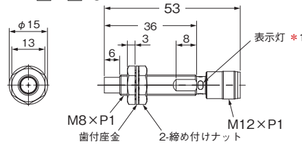
形E2E-X□M□L12-M1
