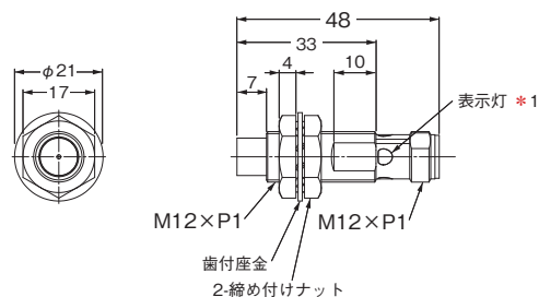
形E2E-X14MD□-M1/-M1G
