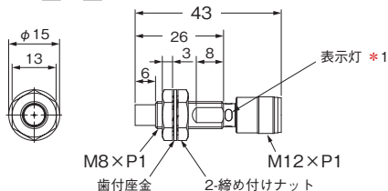
形E2E-X□M□12-M1
