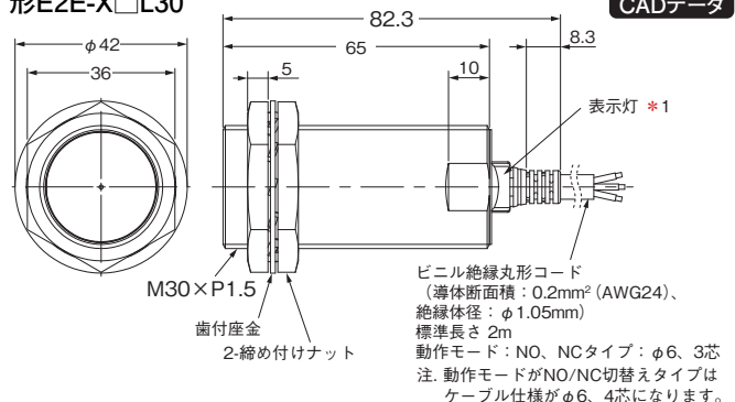
形E2E-X□L30
