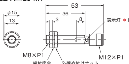
形E2E-X□L12-M1
