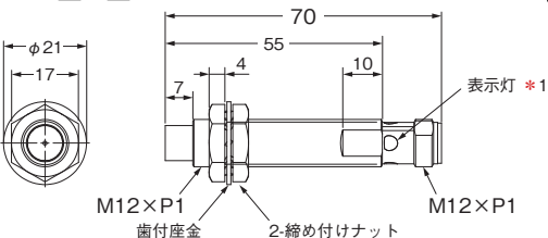
形E2E-X□M□L18-M1
