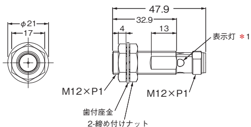
形E2E-X7D□-M1/-M1G
