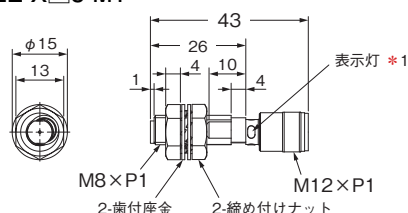
形E2E-X□12-M1
