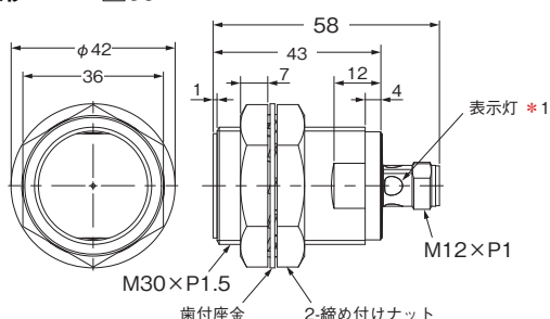
形E2E-X□30-M1
