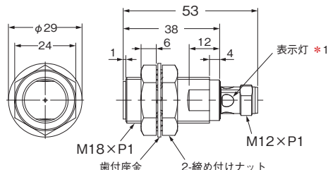
形E2E-X□30-M1
