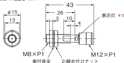
形E2E-X□12-M1
