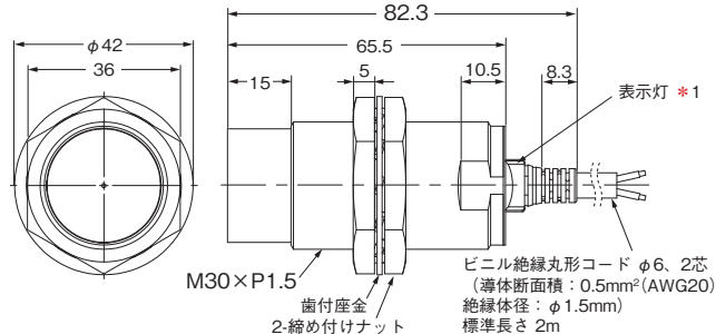
形E2E-X30MD□L
