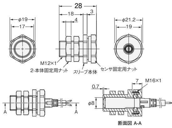
形Y92E-J8S12
