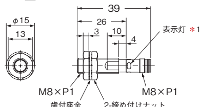
形E2E-X□8-M1
