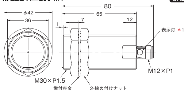
形E2E-X□L30-M1
