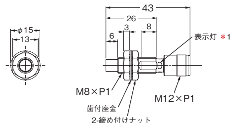
形E2E-X8MD□-M1/-M1G
