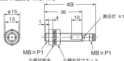
形E2E-X□L8-M1
