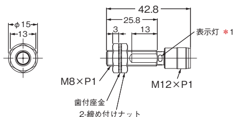
形E2E-X3D□-M1/-M1G
