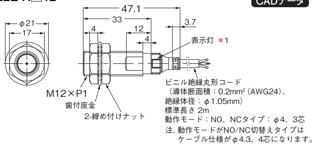
形E2E-X□12
