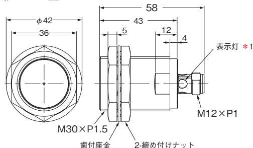
形E2E-X□30-M1
