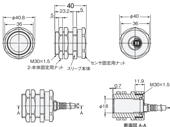
形Y92E-J18S30
