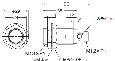
形E2E-X□30-M1
