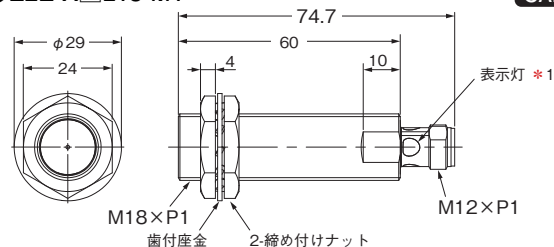
形E2E-X□L30-M1
