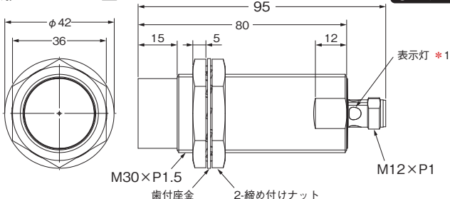
形E2E-X50M□L30-M1
