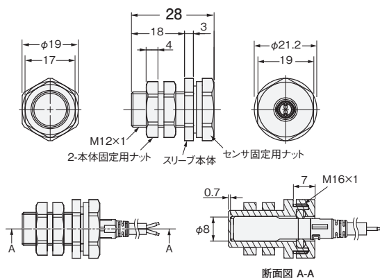
形Y92E-J8S12
