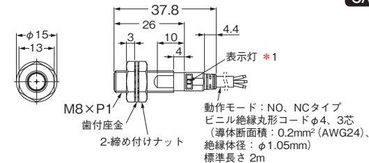
形E2E-X□12
