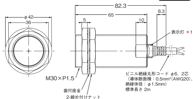
形E2E-X10D□L
