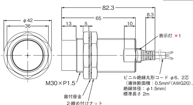
形E2E-X30MD□L
