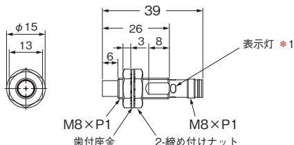
形E2E-X□M□8-M1
