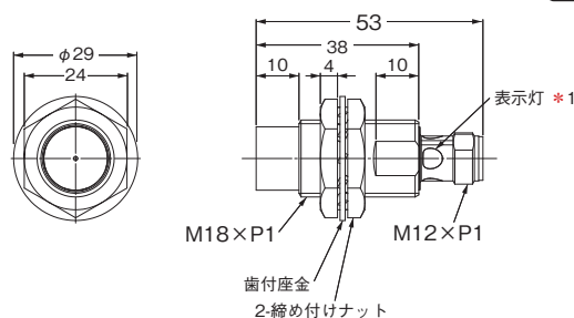
形E2E-X20MD□-M1/-M1G
