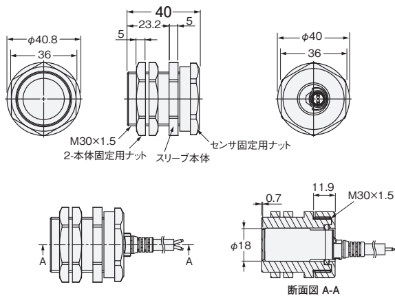
形Y92E-J18S30
