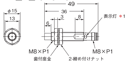
形E2E-X□M□L8-M1
