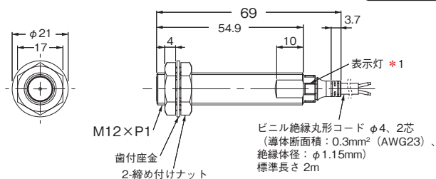
形E2E-X7D□L
