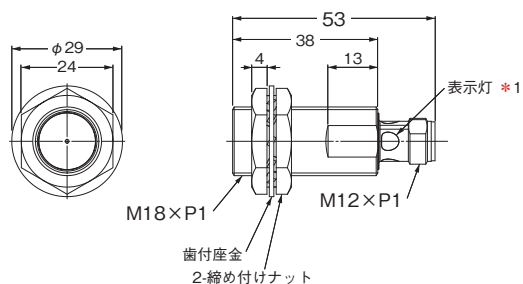
形E2E-X10D□-M1/-M1G
