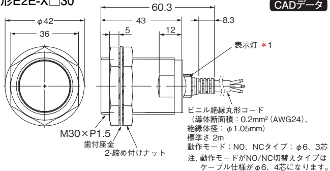
形E2E-X□30
