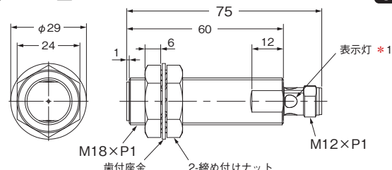
形E2E-X□L30-M1
