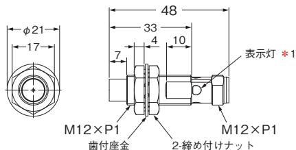
形E2E-X□M□12-M1
