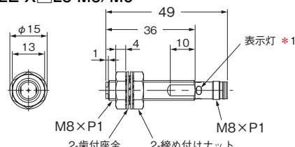
形E2E-X□L8-M1
