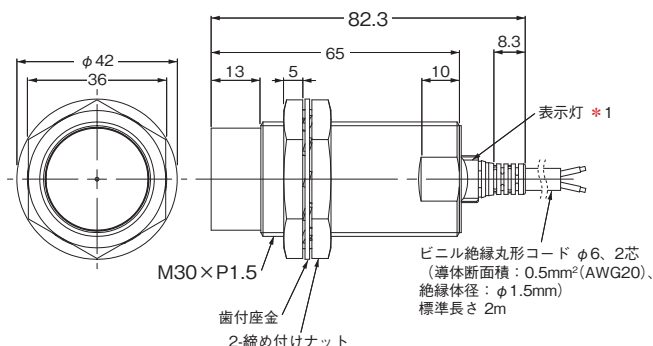
形E2E-X30MD□L
