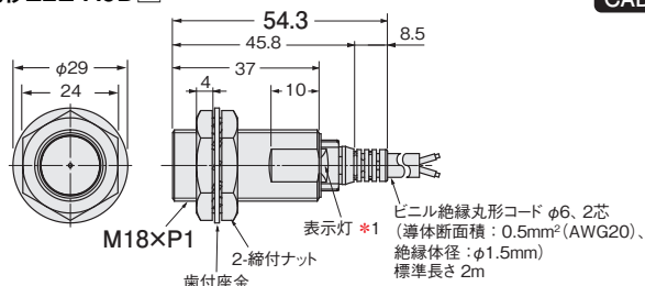
形E2E-X5D□
