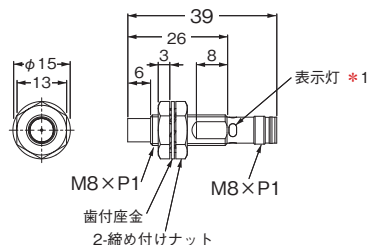
形E2E-X4MD□-M3G
