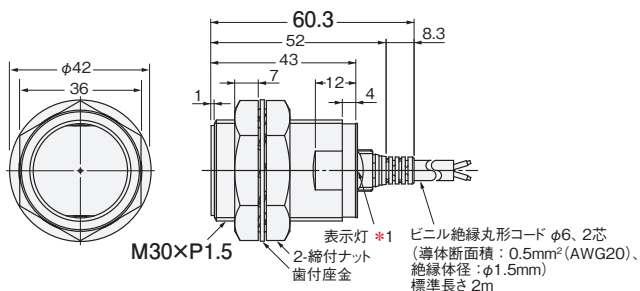
形E2E-X20D□30
