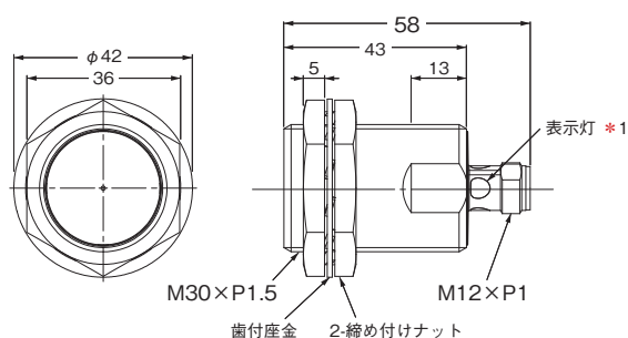
形E2E-X10D□-M1/-M1G
