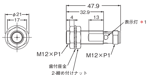
形E2E-X7D□-M1/-M1G
