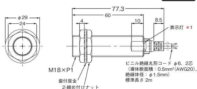
形E2E-X7D□L
