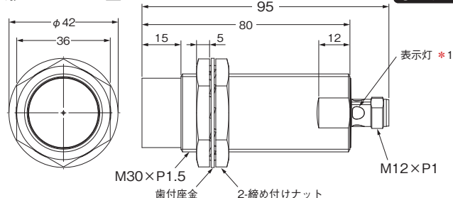
形E2E-X50M□L30-M1
