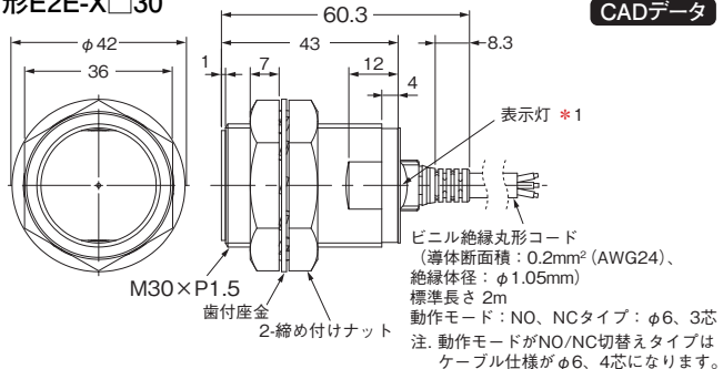
形E2E-X□30
