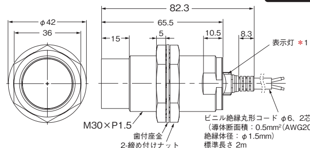
形E2E-X30MD□L
