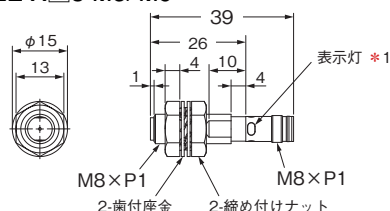
形E2E-X□8-M1
