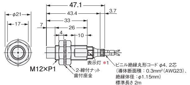
形E2E-X20MD□18
