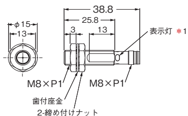
形E2E-X2D□-M3G
