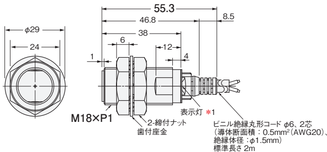
形E2E-X20D□30
