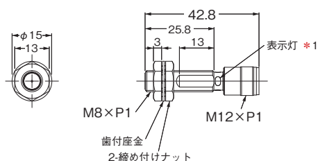
形E2E-X3D□-M1/-M1G
