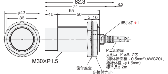
形E2E-X40MD□L30
