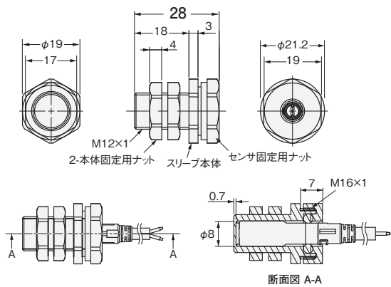
形Y92E-J8S12
