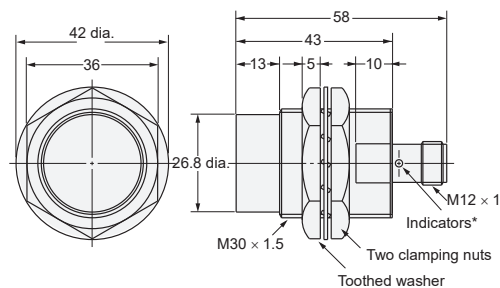
Diagram 16 E2E-X20MD□-M1(G)/E2E-X18ME□-M1/X18MF□-M1
