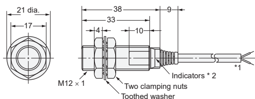
Diagram 3 E2E-X3D□ E2E-X2E□/F□
