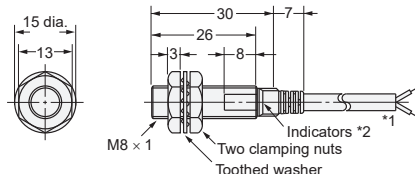
Diagram 1 E2E-X2D□ E2E-X1R5E□/F□
