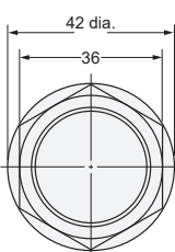
Diagram 22 E2E-X10D□-M1GJ E2E-X10D□-M1J-T E2E-X10D1-M1TGJ E2E-X10D□-M1TGJ-US
