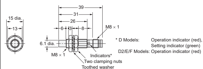
Diagram 18 E2E-X4MD□-M3G/E2E-X2ME□-M3/X2MF□-M3
