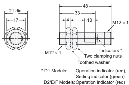
Diagram 11 E2E-X3D□-M1(G) E2E-X2E□-M1/E2E-X2F□-M1
