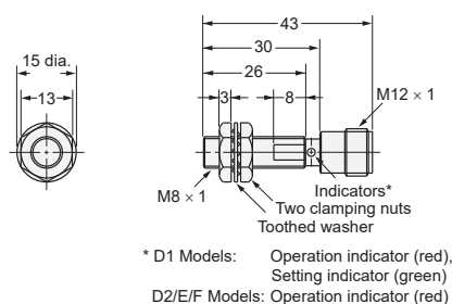
Diagram 11 E2E-X3D□-M1(G) E2E-X2E□-M1/E2E-X2F□-M1
