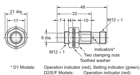
Diagram 12 E2E-X8MD□-M1(G) E2E-X5ME□-M1/E2E-X5MF□-M1
