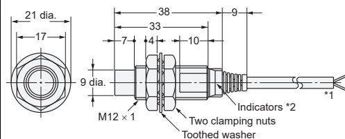
Diagram 4 E2E-X8MD□ E2E-X5ME□/F□
