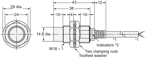
Diagram 6 E2E-X14MD□/E2E-X10ME□/F□
