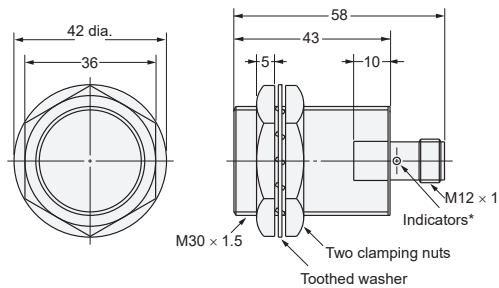
Diagram 15 E2E-X10D□-M1(G)/E2E-X10E□-M1/X10F□-M1
