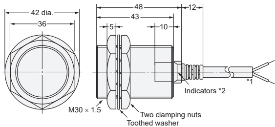
Diagram 7 E2E-X10D□/E2E-X10E□/F□
