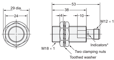
Diagram 13 E2E-X7D□-M1(G)/E2E-X5E□-M1/X5F□-M1
