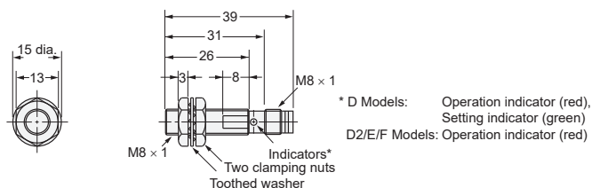
Diagram 17 E2E-X2D□-M3G/E2E-X1R5E□-M3/X1RF□-M3
