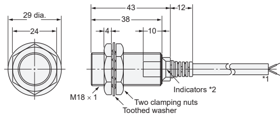
Diagram 5 E2E-X7D□/E2E-X5E□/F□
