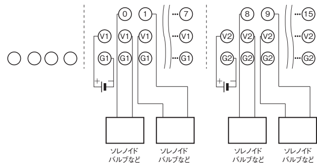
形DRT2-MD16TA (NPN対応)
