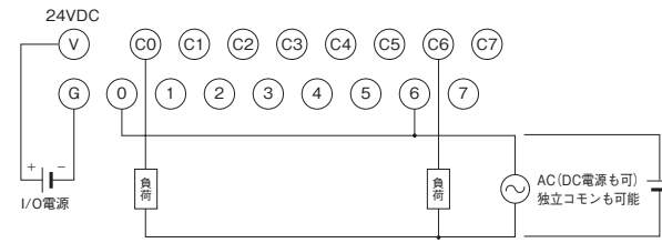
形GT1-ROP08/形GT1-FOP08
