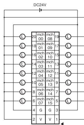
形DRT2-OD16ML (X) (NPN対応)
