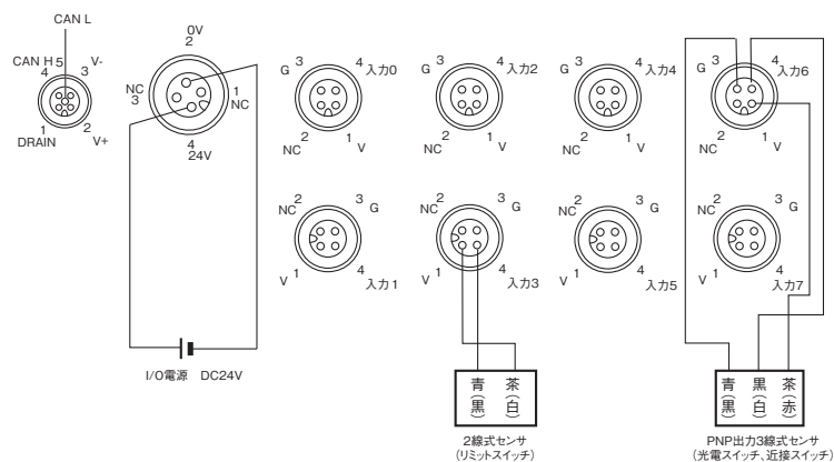
形DRT2-ID08CL-1 (PNP対応)
