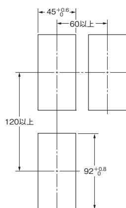
パネル加工寸法
