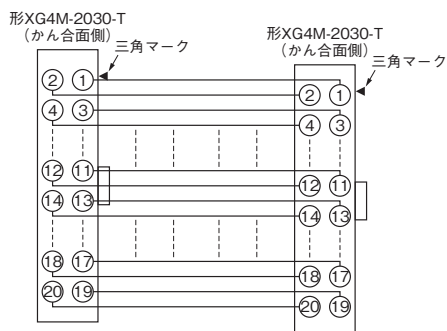
形DRT2-ID16MLX(-1)/形DRT2-OD16MLX(-1)付属コネクタ付ケーブル配線図
